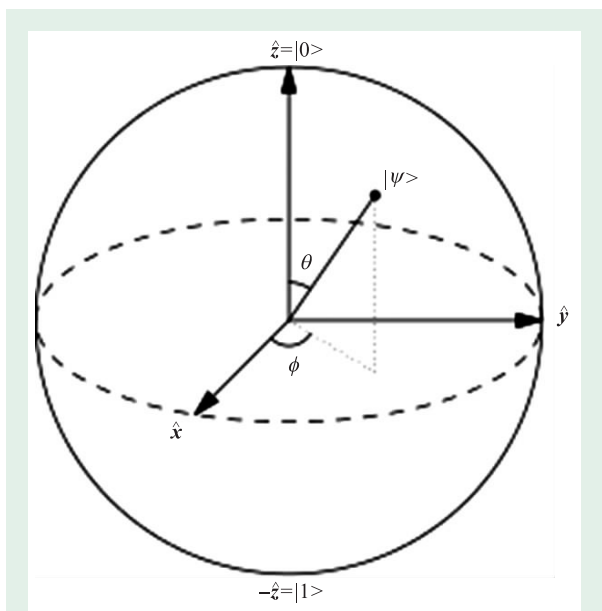
图2 表示量子比特的 Bloch 球，球面代表了一个量子比特所有可能的取值
