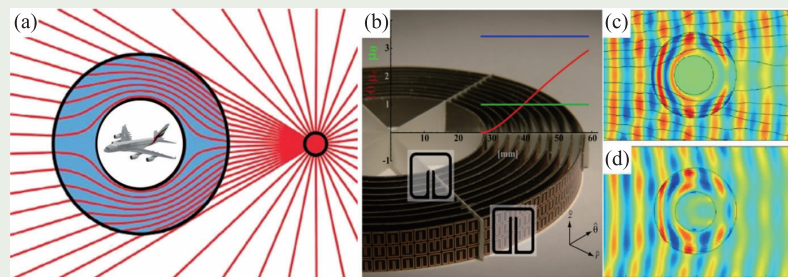
图4 全向隐身技术 [1, 2] (a)探测波绕射的隐身原理；(b)窄带微波频段简化参数隐身结构实物图；(c)简化参数隐身结构的仿真隐身效果；(d)实验测量的电场强度分布
