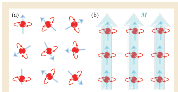
图3 自发磁化的示意图 (a)磁矩随机排布，无自发磁化；(b)磁矩有序排布，产生自发磁化
