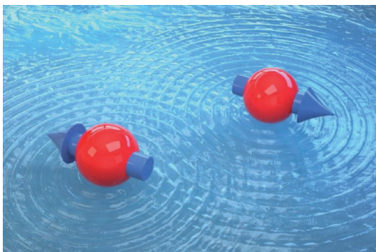
图1 康普顿的设想：“自旋”及其产生的磁场
