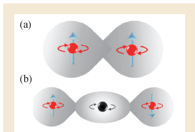
图4 交换相互作用的示意图 (a)直接交换相互作用；(b)间接交换相互作用
