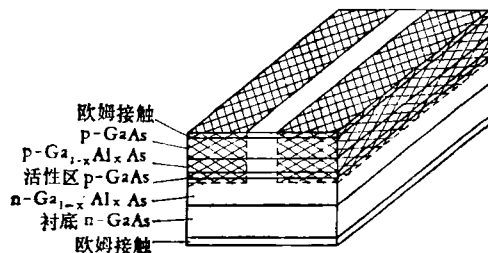
图 1 条形砷化镓双异质结激光二极管的结构
