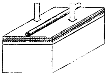
图 2 用质子轰击外延片的示意图。箭头表示质子束的轰击方向。打斜线的区域是被质子轰击后变成高阻的部分。被钨丝遮住的部分就是条形区域
