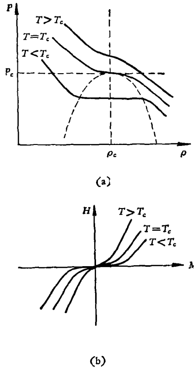
图3 状态方程的等温线 (a) 液体；(b) 铁磁体
