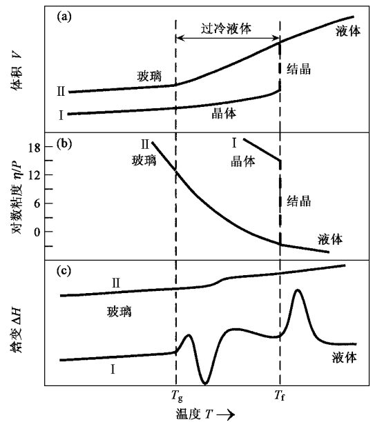
图1 液体(熔体)从高温冷却到室温所经历的结晶(a)或(b)中的途径I,或玻璃化转变过程(a)或(b)中的途径II,和从低温将玻璃加热到高温熔化或重新转变为液体(c)中的途径I,或经过晶化过程到达平衡的液相,途径II为无晶化过程的转变. T_f 是平衡的结晶温度, T_g 为玻璃化转变温度.
