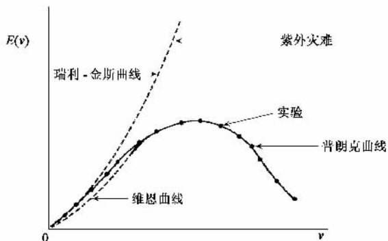
图1 黑体辐射能量密度 E(\nu) 随频率 \nu 变化
