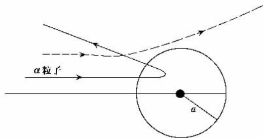
图2 卢瑟福的 \alpha 粒子对原子的散射
