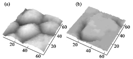
图2 在5%晶格失配下,初始为10个单层厚的平坦薄膜退火模拟所得的表面构形 (a)温度为1000K,时间为100 \mu\text{s} (b)600K,0.25s
