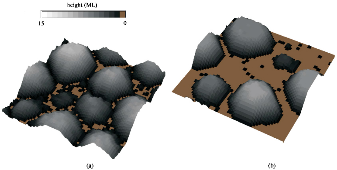
图1 在8%晶格失配下,模拟薄膜沉积所得的表面构形 (a)温度为1000K,生长速率为20000单层每秒 (b)600K,10单层每秒
