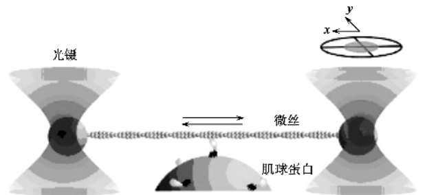
图 3 双光镊测量微丝与肌球蛋白作用力与运动步幅的示意图
