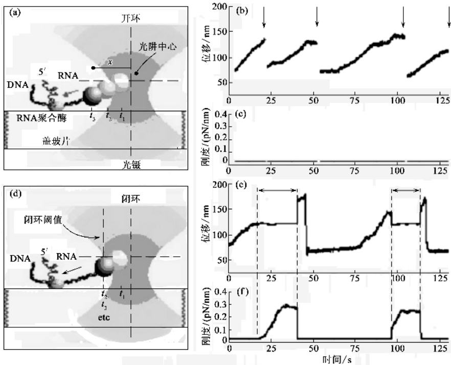
图4 (a,d)分别为光镊在开环与闭环条件下,测量RNA聚合酶转录速度与力的示意图(b,c)为开环条件下测得的小球的位移以及光阱刚度随时间的变化关系曲线(e,f)对应于闭环条件
