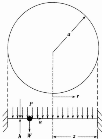
图2 A sketch(草图、简图)
