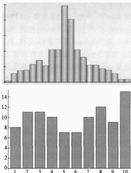
图3 Histogram (叙事图). 长条形的画法根据要表现的内容是有讲究的
