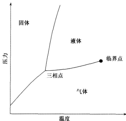
图 5 物质的相图 (phase diagram): 这里描绘的是物质的状态随温度和压力的变化
