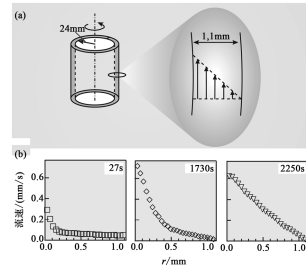
图 1 一组典型的速度分布实验结果 (a) 库埃特圆筒的几何结构; (b) 一组典型的速度分布
