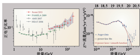
图 3 宇宙线最新结果 (a) PAMELA 和 Fermi 卫星能谱仪测到的正电子比率在 10—200GeV 能区令人惊讶地持续上升; (b) 由 Pierre Auger 观测站测量到的 10^{18} eV 能量以上宇宙线能谱, 在 3 \times 10^{19} eV 附近的陡降可能是预计的 Greisen—Zatsepin—Kuzmin (GZK) 截断。曲线和直线是对数据的不同拟合
