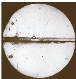
图2 一张有历史意义的云雾室照片,由卡尔·安德森1932年拍摄.照片显示一个可能来自于宇宙线簇射的正电荷粒子,从上面进入,被云雾室的横向磁场打弯,最后在铅板中丢失了能量.这是首次看到保罗·狄拉克1928年预言的正电子
