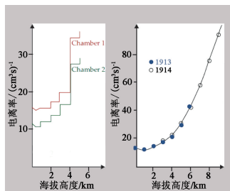
图1 大气电离率随海拔高度的变化函数 (a)由赫斯于1912年8月7日测得;(b)由科赫斯特于1913年测得
