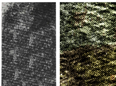
图9 金单晶格子像(左图分辨率为 2.04\text{ \AA} (200面);右图分辨率为 1.43\text{ \AA} (220面))
