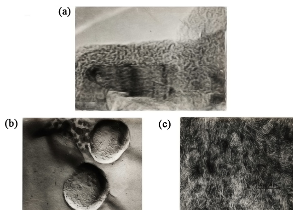
图8 (a)石墨化碳黑碳化粒子(分辨率为 4\text{ \AA} ,总放大倍数为 3,000,000\times ,高压 100\text{ kV} );(b)砂眼衣原体(放大倍数为 90,000\times );(c)聚对苯二甲酸乙二醇酯脂片晶
