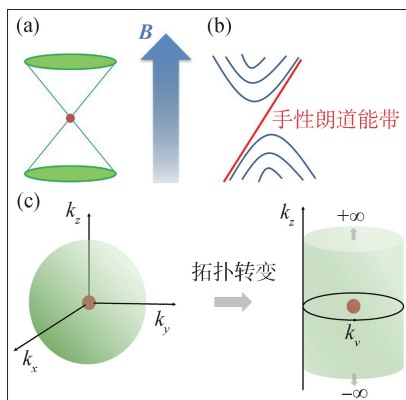
(a)单个外尔点加磁场；(b)朗道能带结构包含一条手性能带；(c)拓扑费米点的拓扑荷与映射得到的陈绝缘体陈数相等
